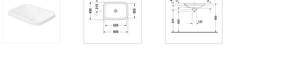
Умывальник встраиваемый, 037260
