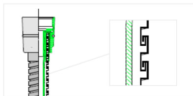
DOPPIA AGGRAFFATURA - DOUBLE INTERLOCK
