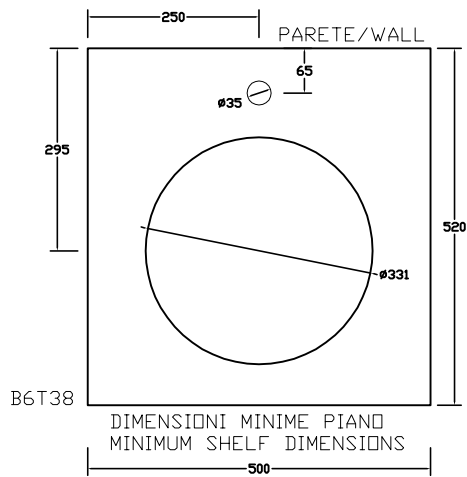
RUBINETTO SU PIANO SHELF TAP
