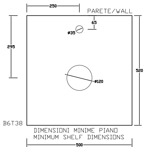
RUBINETTO SU PIANO SHELF TAP
