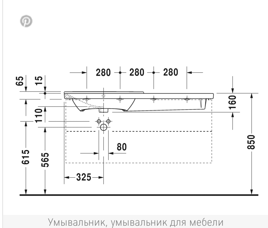
Умывальник, умывальник для мебели асимметричный, 233312
